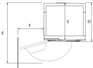
WAND DRAUFSICHT
